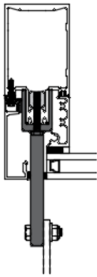
P6942 - 400CW/T Vertical End Jamb
