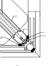
7B CORNER OPTIONAL
