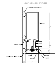
4 STANDARD TUBULAR JAMB
