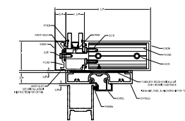
9A STANDARD TRANSOM
