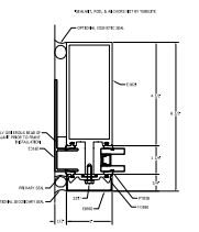
4C OPTIONAL TUBULAR JAMB WITH 7\"/>
