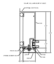
4A OPTIONAL OPEN BACK JAMB
