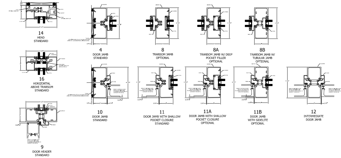
DOOR DETAILS
